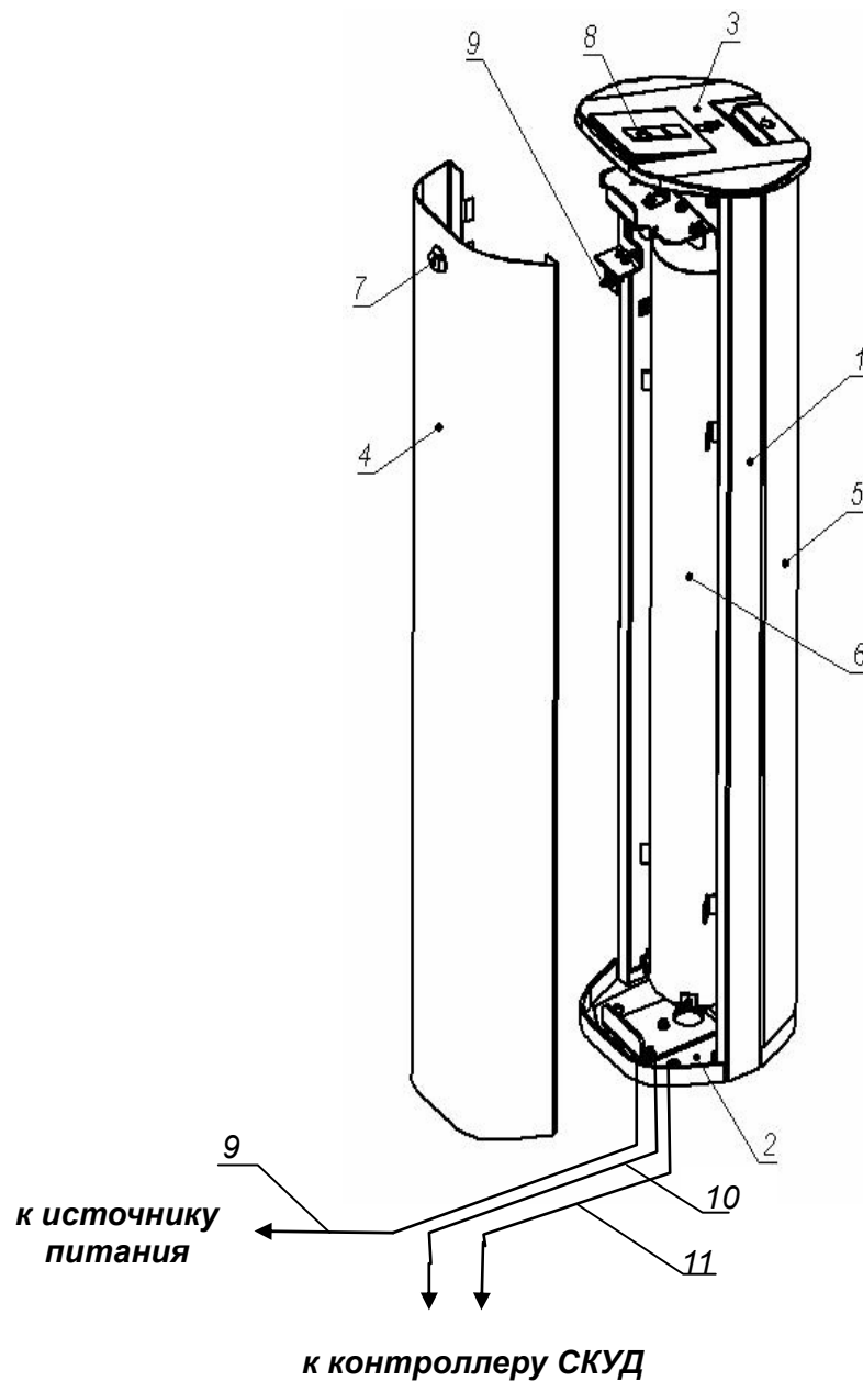
Рисунок 1 – Устройство картоприёмника:
