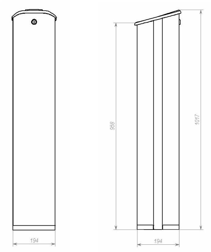
Рисунок 3 – Габаритные размеры картоприёмника
