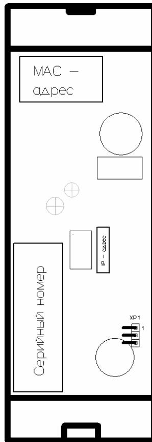
Рисунок 1 - Внешний вид тыльной стороны контроллера PERCo-CL05
