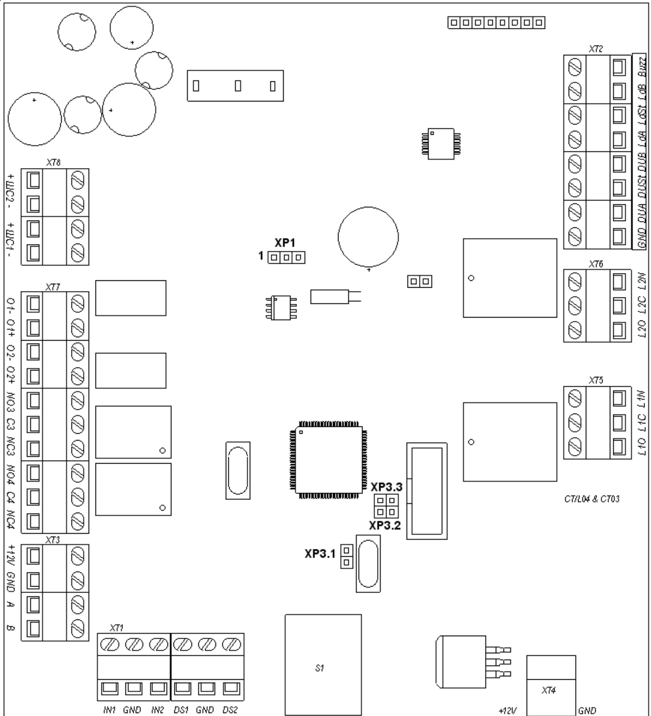
Рисунок 1 - Внешний вид печатной платы контроллера PERCo-CT/L04 Цоколевка разъемов
