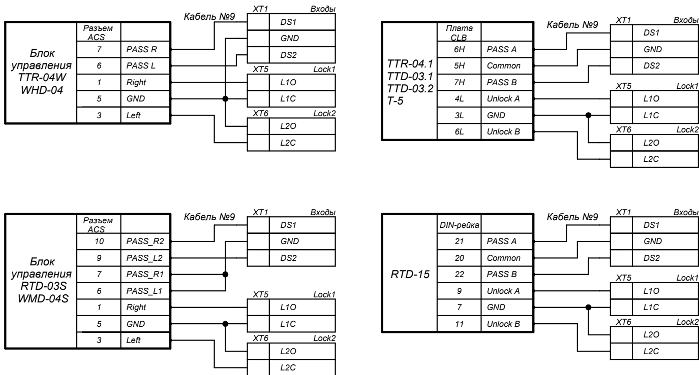
Рисунок 4 – Схема подключений ИУ в варианте «управление турникетом с УИ»
