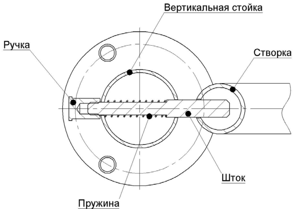
Рисунок 14 – Установка штока стопорного узла
