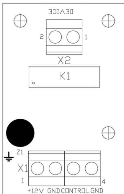
Рисунок 8 – Внешний вид платы.
