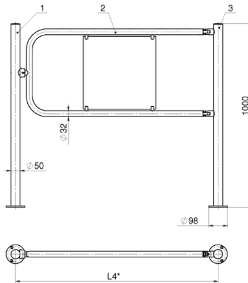
Рисунок 6 – Автоматическая поворотная секция ограждения:
