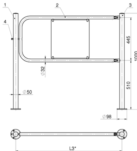
Рисунок 5 – Механическая поворотная секция ограждения типа:
