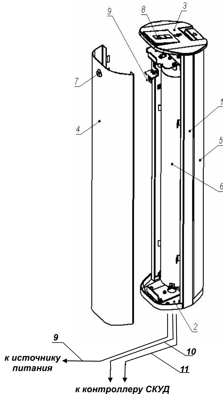
Рисунок 1 – Устройство картоприёмника:
